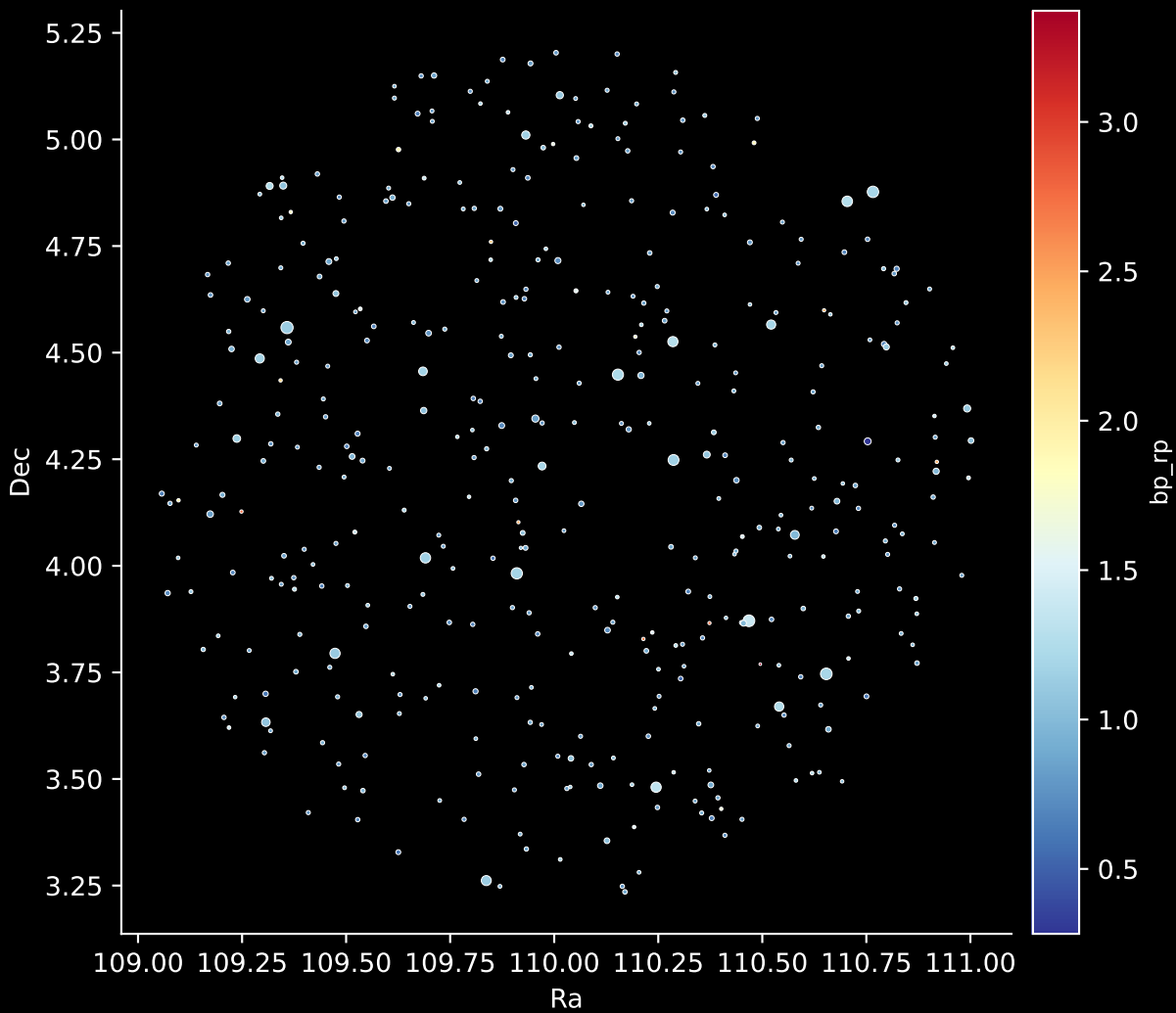
GALAH DR4 Field: [6697] Stars: 394
