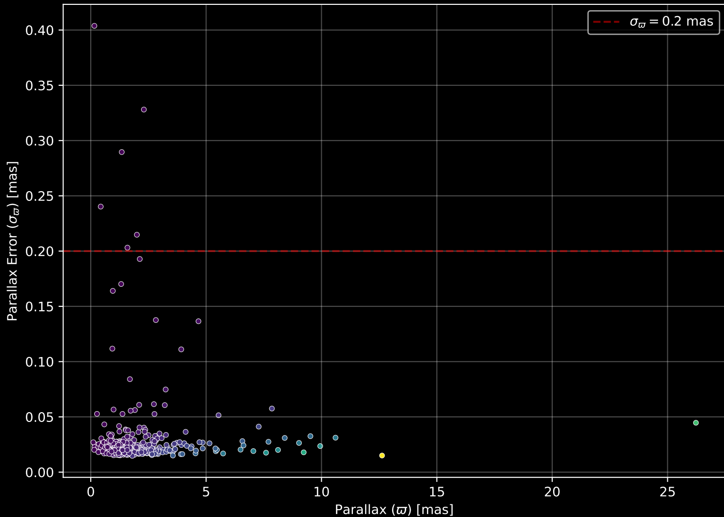
GALAH DR4 Field: [6697] Parallax Quality (n= 394)
