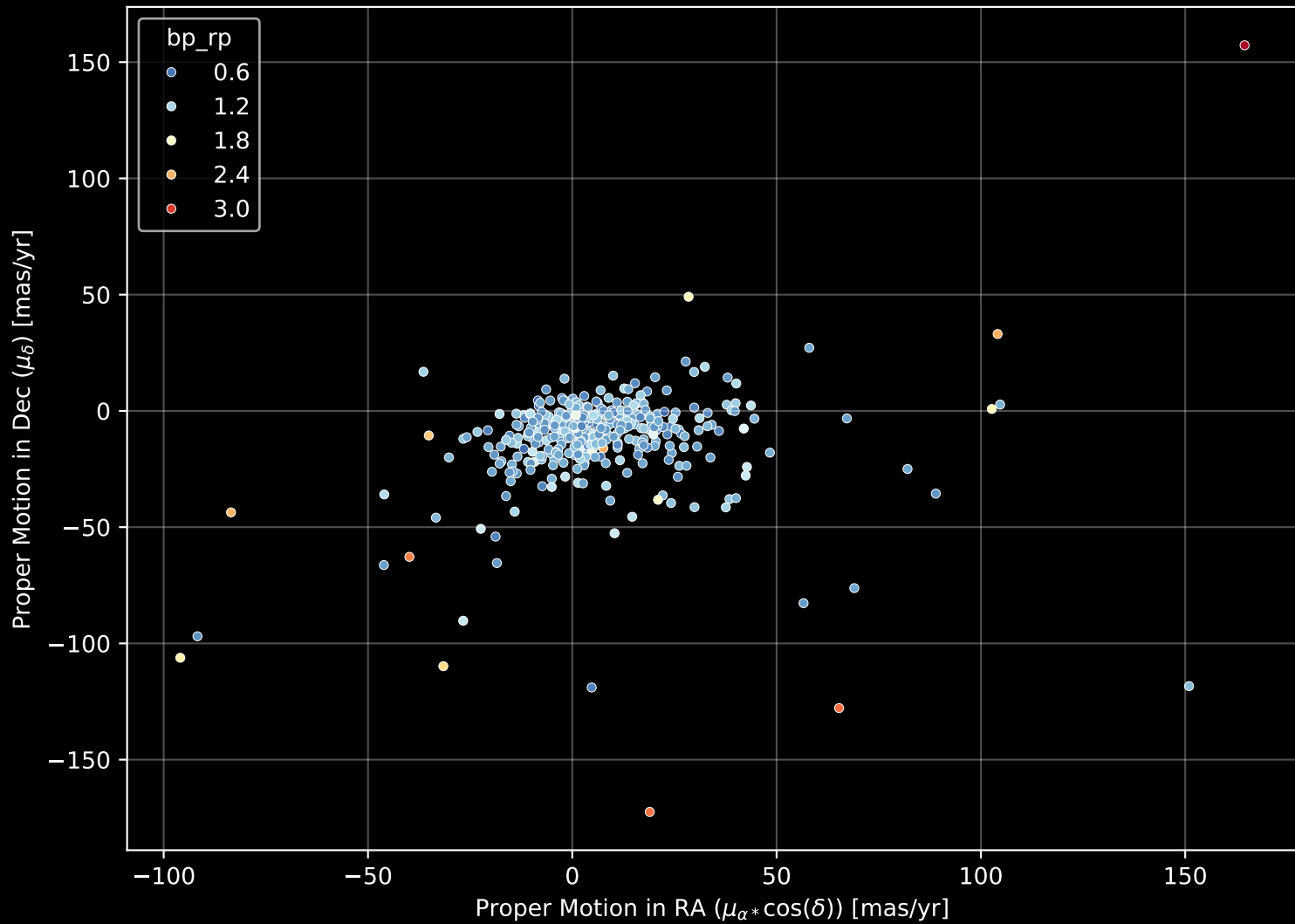
GALAH DR4 Field: [6697] Proper Motion Diagram (n= 394)
