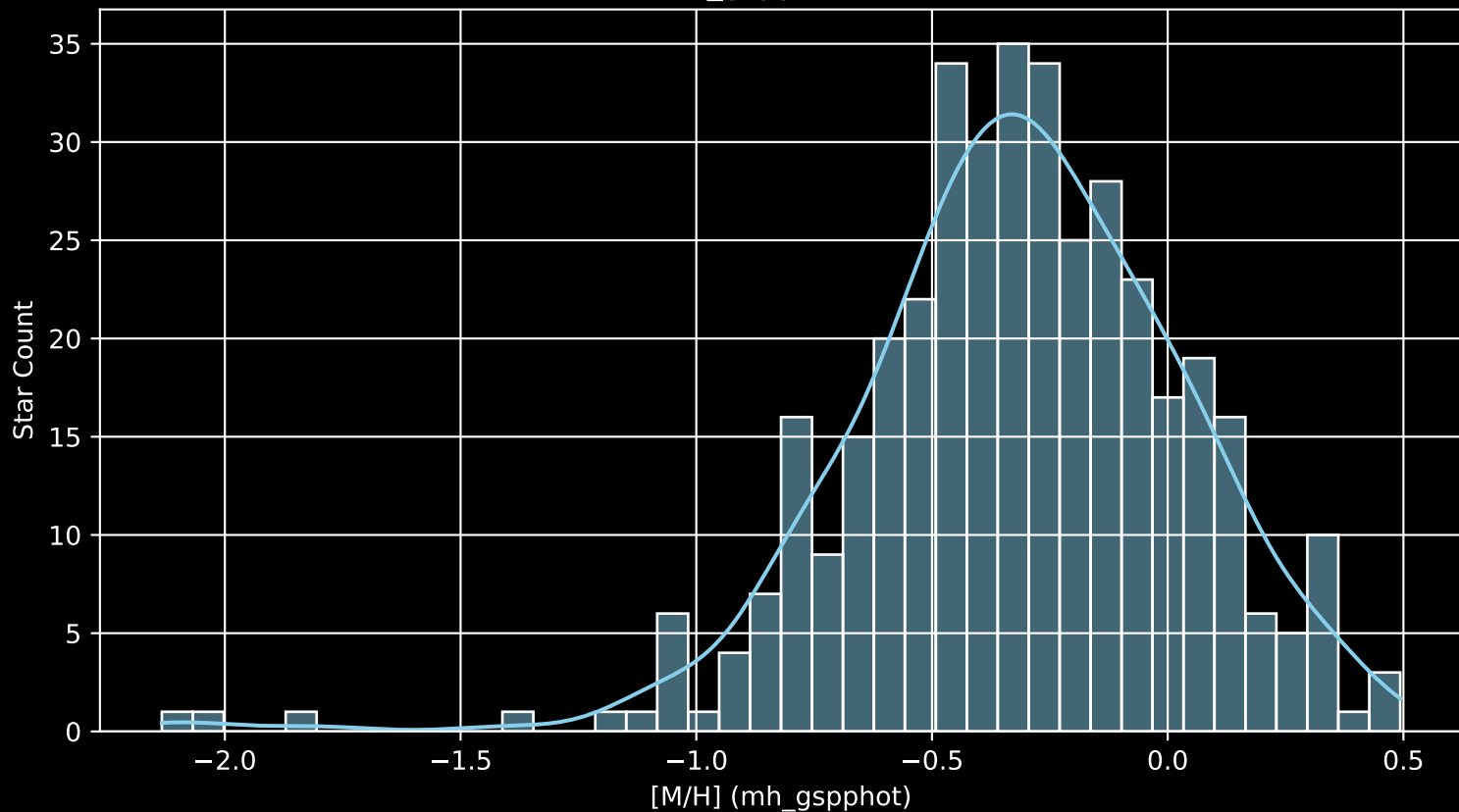
GALAH DR4 Field: [6697] [M/H] (mh_gspphot) (n= 392)
