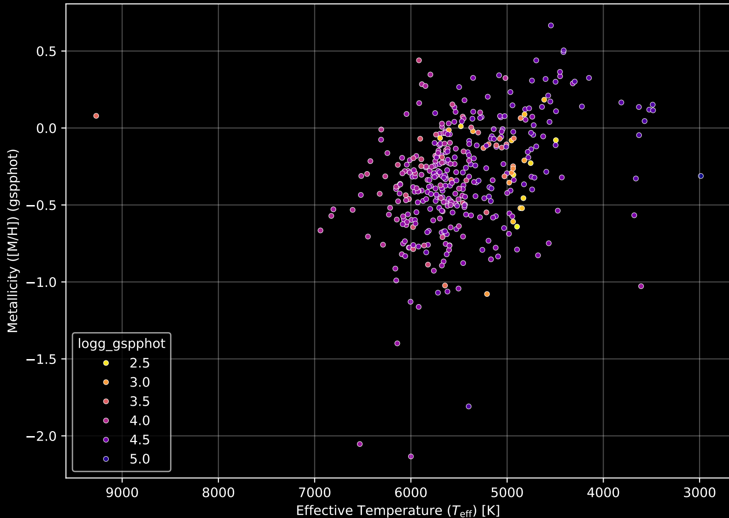
GALAH DR4 Field: [6697] Stellar Population Parameters (n= 394)
